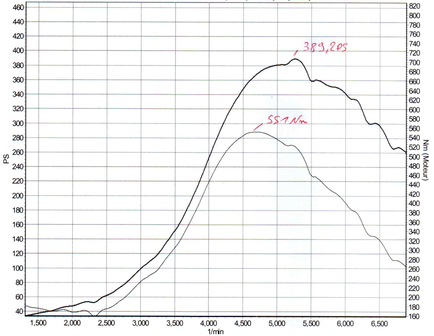
Puissance-max Puissance Moteur (corr.) / Couple (corr.) / Vitesse
